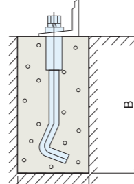
基礎穴寸法
