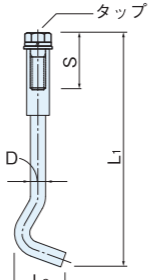
基礎ボルト寸法
