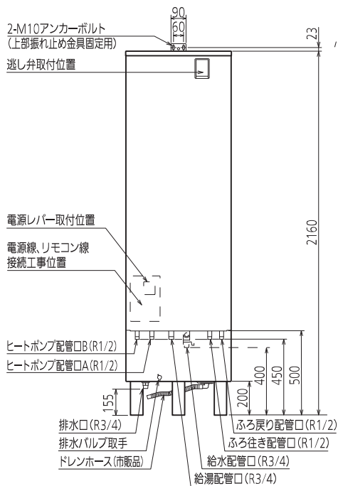
正面図
