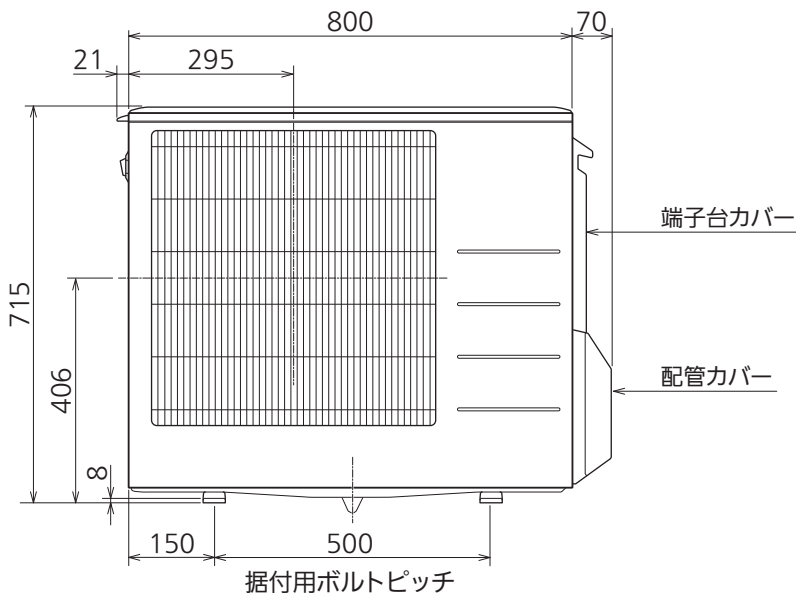
正面図
