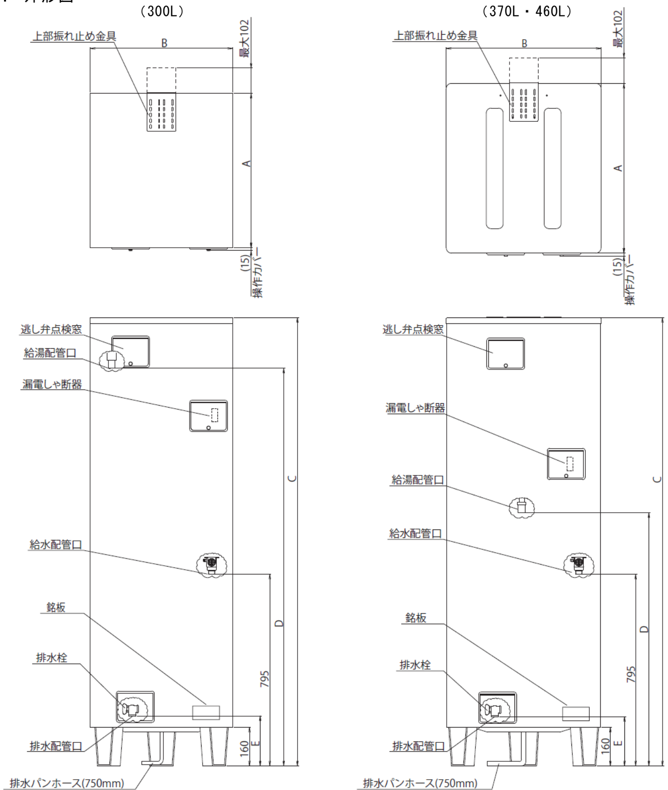
各部の寸法
