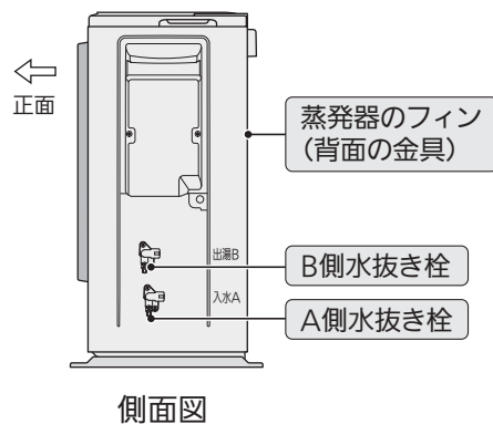
〈配管カバーを外した図〉
