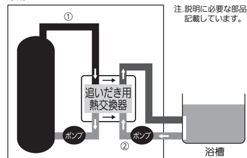
貯湯ユニット
